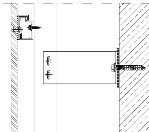
freies Lager (Gleitpunkt)
