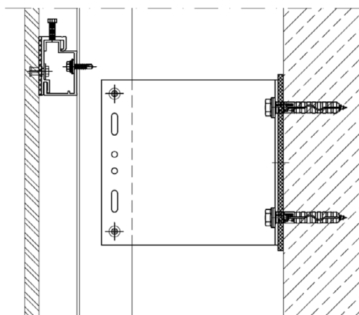
festes Lager (Festpunkt)
