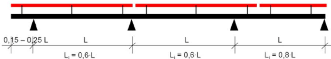
Bild 7: Ideelle Stützweite
