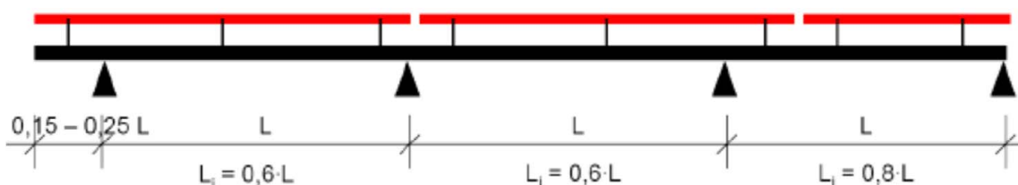
Bild 7: Ideelle Stützweite
