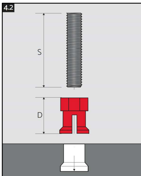
a) Einführen der Hülse in die Hinterschnittbohrung und Eindrehen des Gewindestiftes in die Hülse
