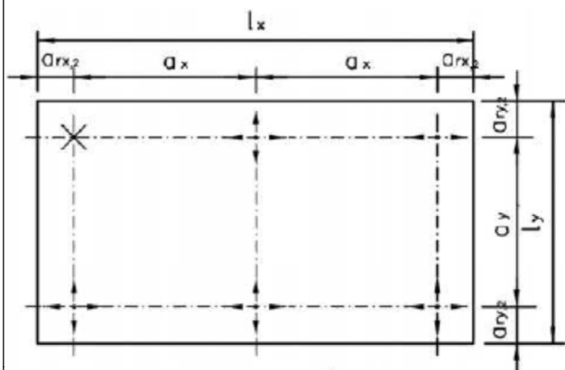
Bild 4: Fassadenplatte mit 6 Agraffen – Lagerungsart 3
