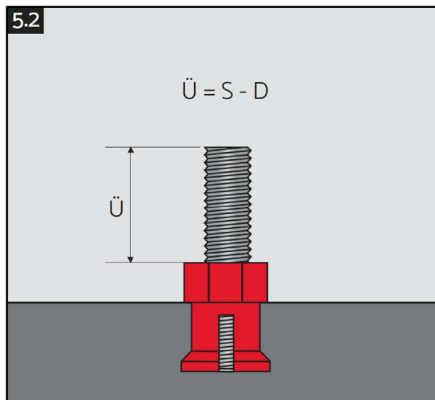
b) eingebauter Hinterschnittanker
