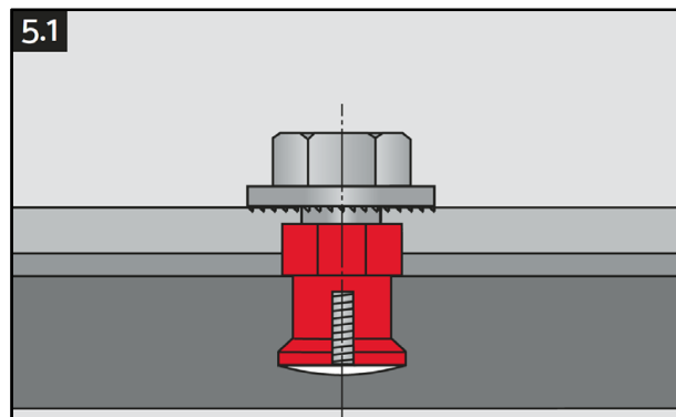
b) eingebauter Hinterschnittanker
